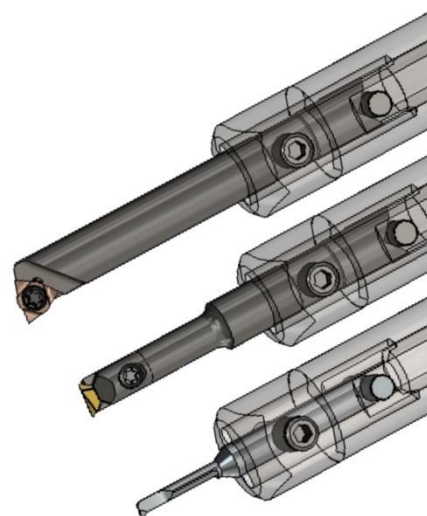
System MINIFIX mit V-Nut Fixierung
